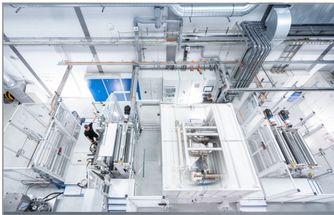
Rolle-zu-Rolle Anlage atmoFlex 1250 für die Sterilisation großflächige Textilien oder anderer flexibler Materialien
